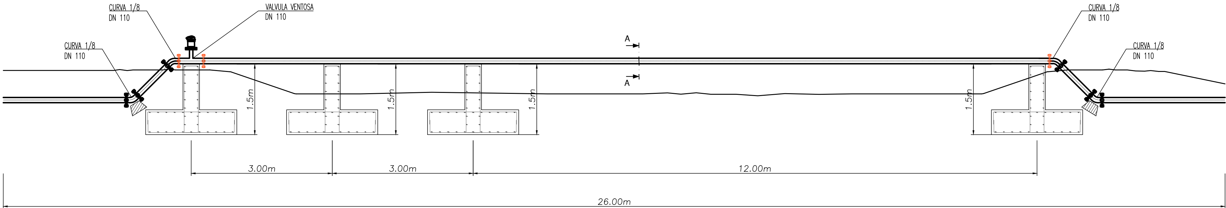
VISTA LATERAL ATRAVIESO AEREO N°2 ESCALA 1 : 50
