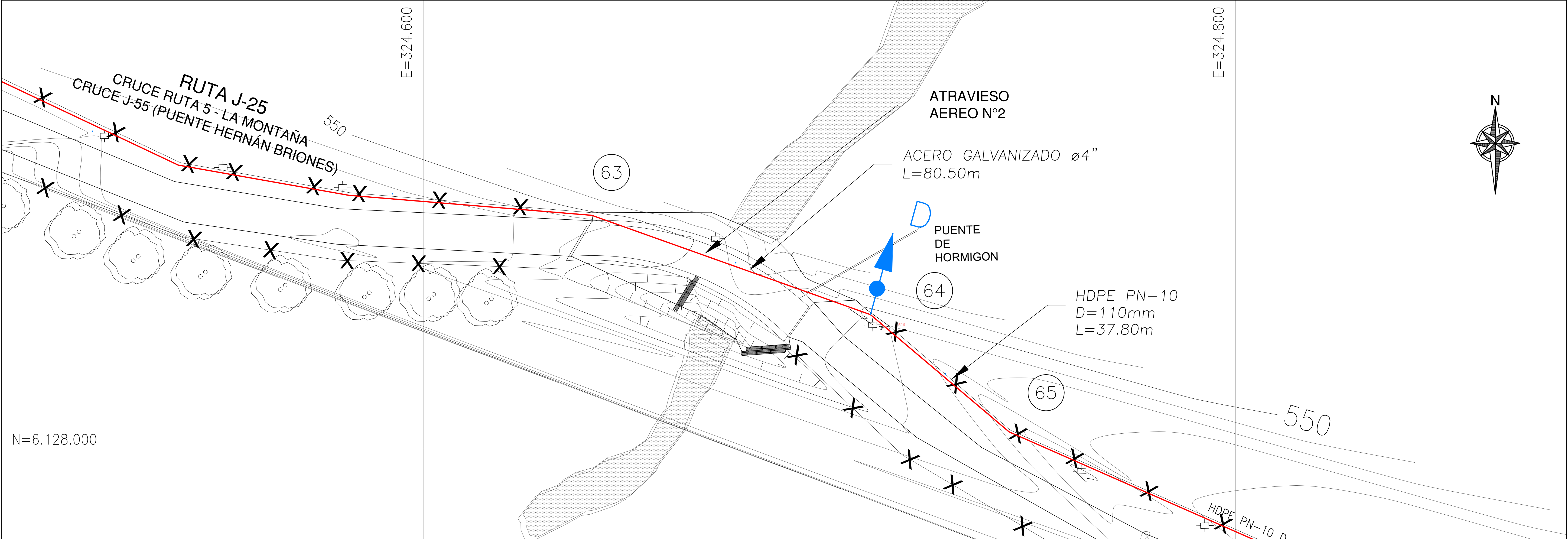
PLANTA ATRAVIESO N°2 ESCALA 1 : 500
